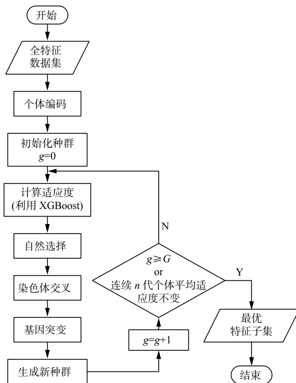
图 2 GA-XGBoost 算法
